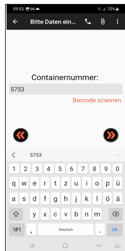
Eingabe Containernummer
