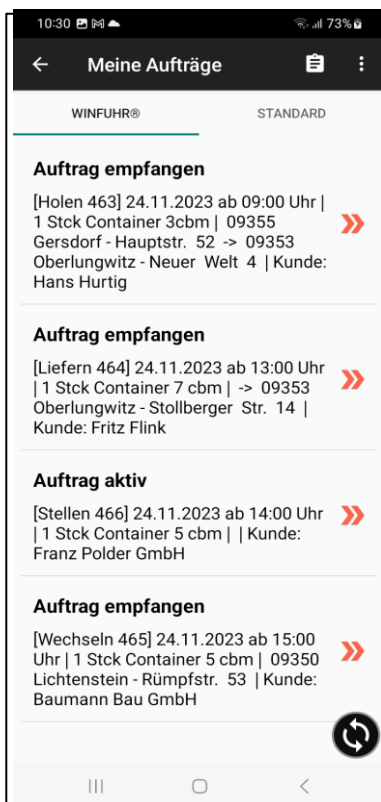
Auftragsliste Fahrer
